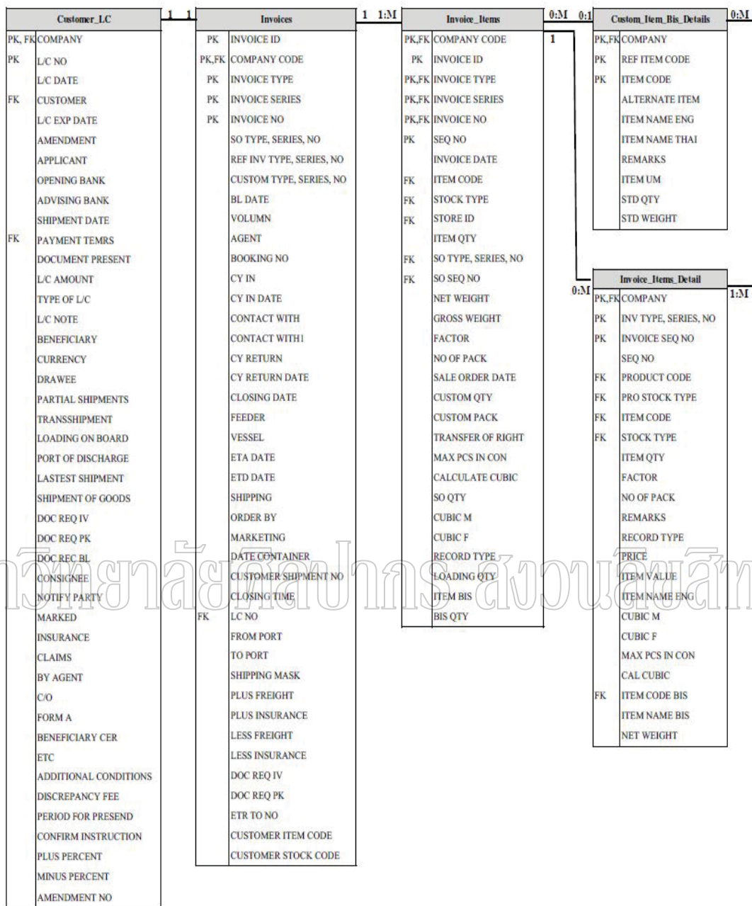
ภาพที่ 12 ER Diagram 3
