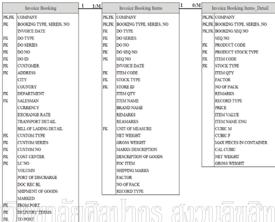
ภาพที่ 13 ER Diagram 4
