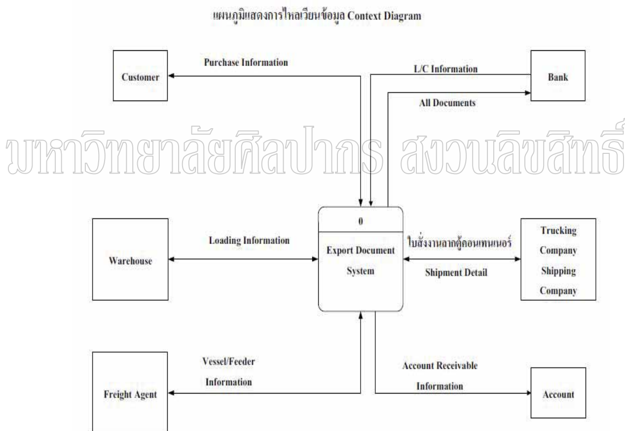
ภาพที่ 7 Context Diagram
