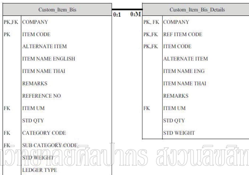
ภาพที่ 10 ER Diagram 1
