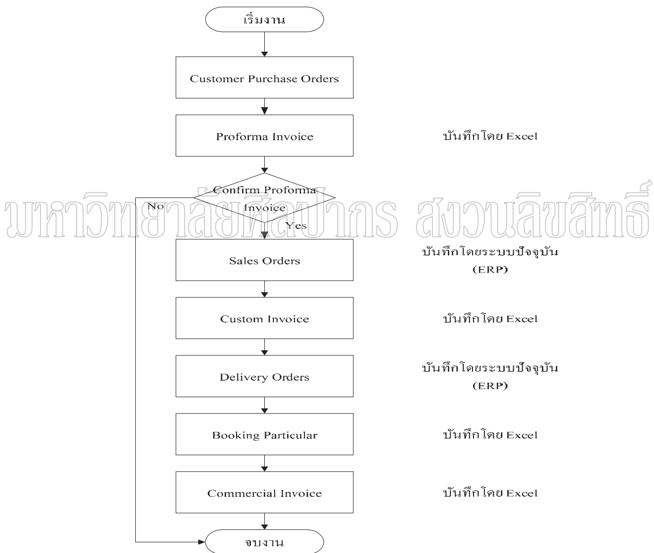
ภาพที่ 2 แสดงการทำงานของระบบปัจจุบัน
