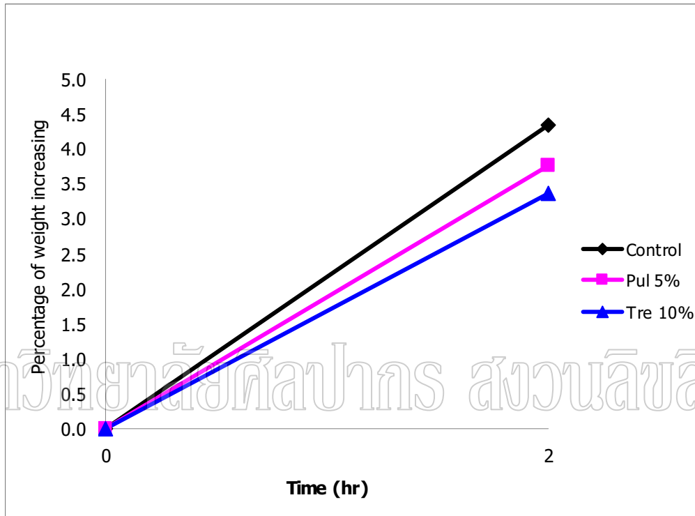
ภาพที่ 13 ผลการดูดซับความชื้นที่ความชื้นสัมพัทธ์ 70 % นาน 2 ชั่วโมง
