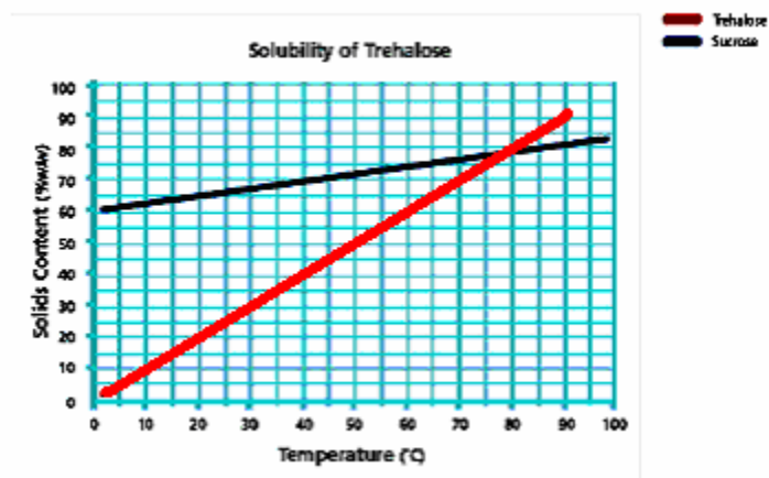
ภาพที่ 5 การละลายของทรีฮาโลสที่อุณหภูมิต่างๆ
