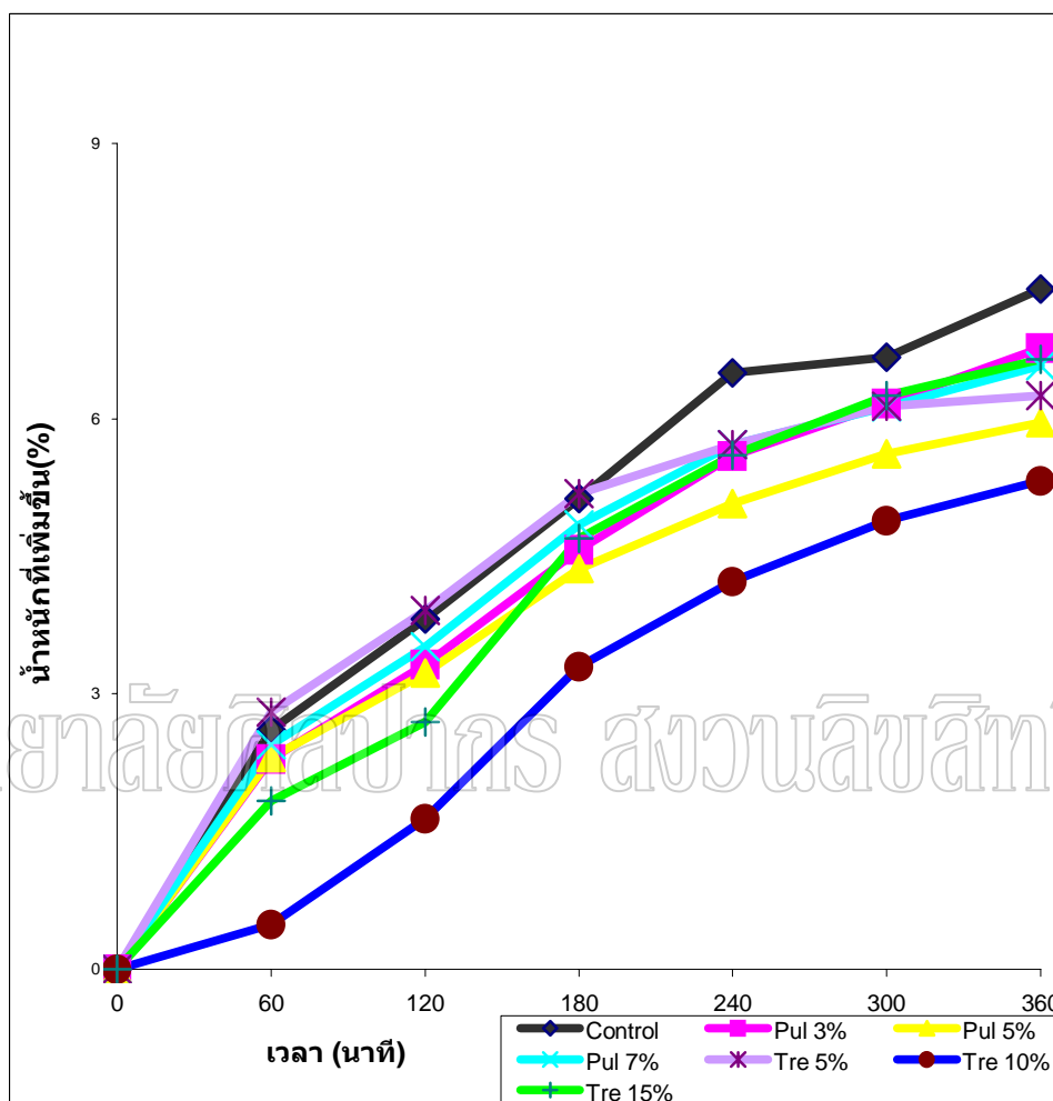
ภาพที่ 10 ผลการดูดซับความชื้นที่ความชื้นสัมพัทธ์ 70 % ของขนมซึ่งเคลือบด้วยสารเคลือบสูตรควบคุม(control) และสูตรการใช้ที่มีพัลลูแลน (Pul) 3, 5, 7 % และ ทรีฮาโลส (Tre) 5, 10, 15 % ตามลำดับ
