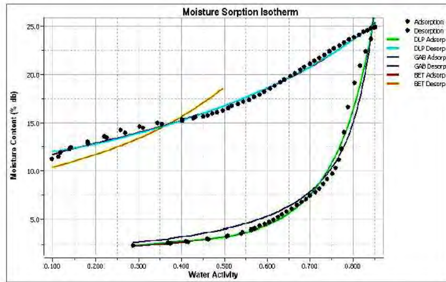
ภาพที่ 17 แสดงค่าความสัมพันธ์ระหว่างความชื้น (ร้อยละน้ำหนักแห้ง)และปริมาณน้ำอิสระของขนมข้าวอบกรอบของชุดผลิตภัณฑ์ที่เคลือบด้วยสารเคลือบสูตรที่ผสมทรีฮาโลส 10 %
