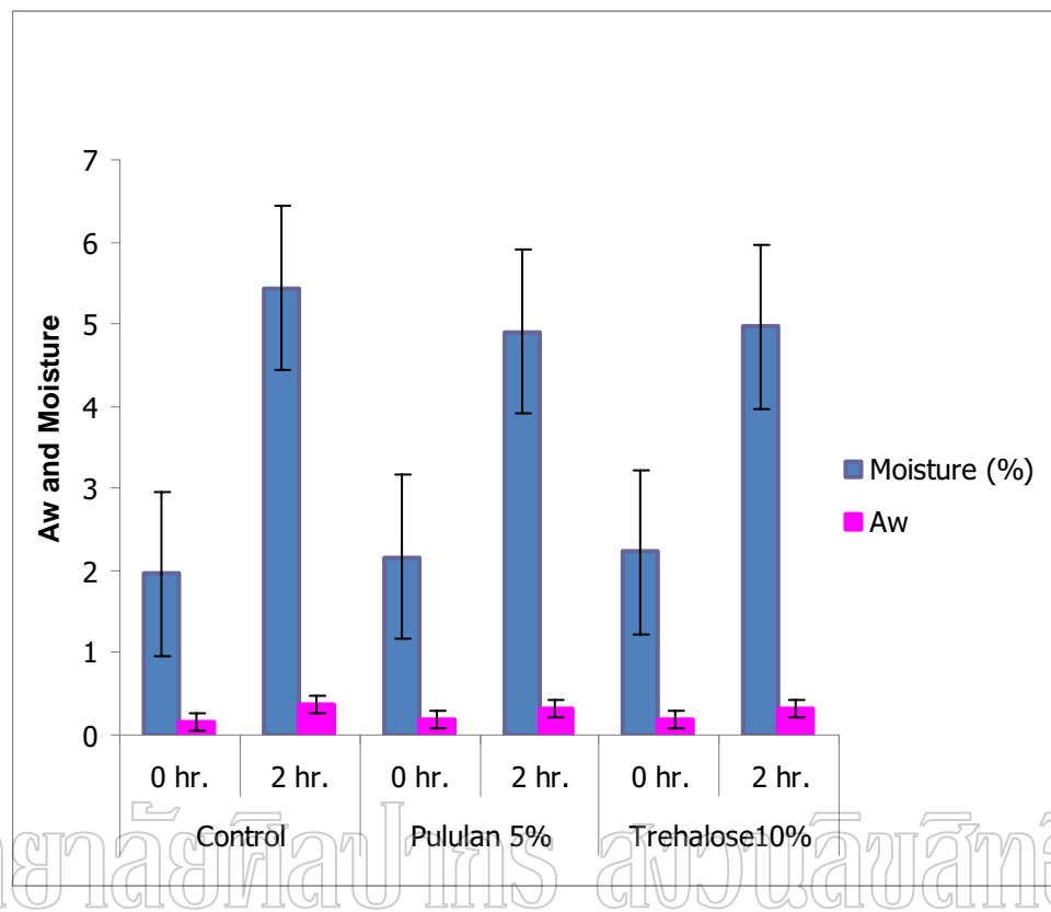
ภาพที่ 14 ความชื้นและค่า a_w ของขนมข้าวอบกรอบสูตรควบคุม สูตรผสมพัลูลาน 5% และ สูตรผสมทรีฮาโลส 10% หลังเก็บในตู้ที่มีความชื้นสัมพัทธ์ 70 % นาน 2 ชั่วโมง
